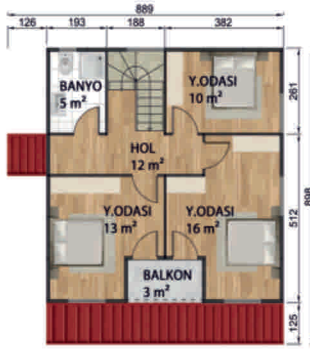
1. Kat Planı 56 \text{ m}^2 + 3 \text{ m}^2 Balkon = 59 \text{ m}^2
