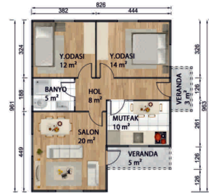
Tek Katlı Prefabrik Konut 69 m 2 + 8 m 2 Veranda
