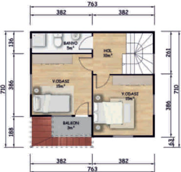
1. Kat Planı 45 m 2 + 3 m 2 Balkon = 48 m 2
